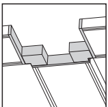
UNIÓN TIPO T / JOINT TYPE T / UNION TIPO T / GIUNTO TIPO T / VERBINDUNG TYP T
